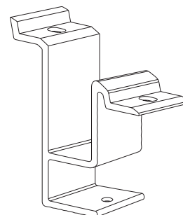
Takstolskonsol 27°
